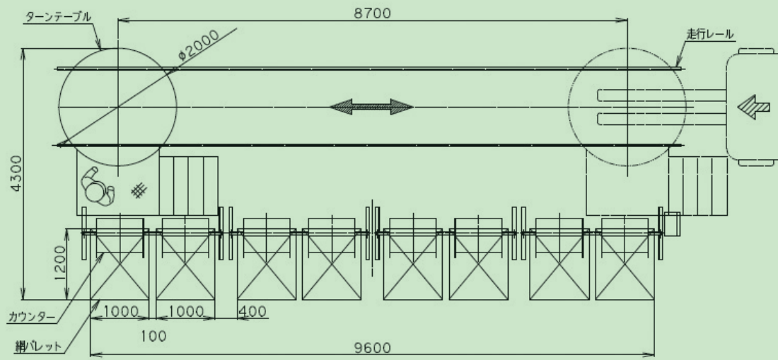
テーブル移動台車方式
