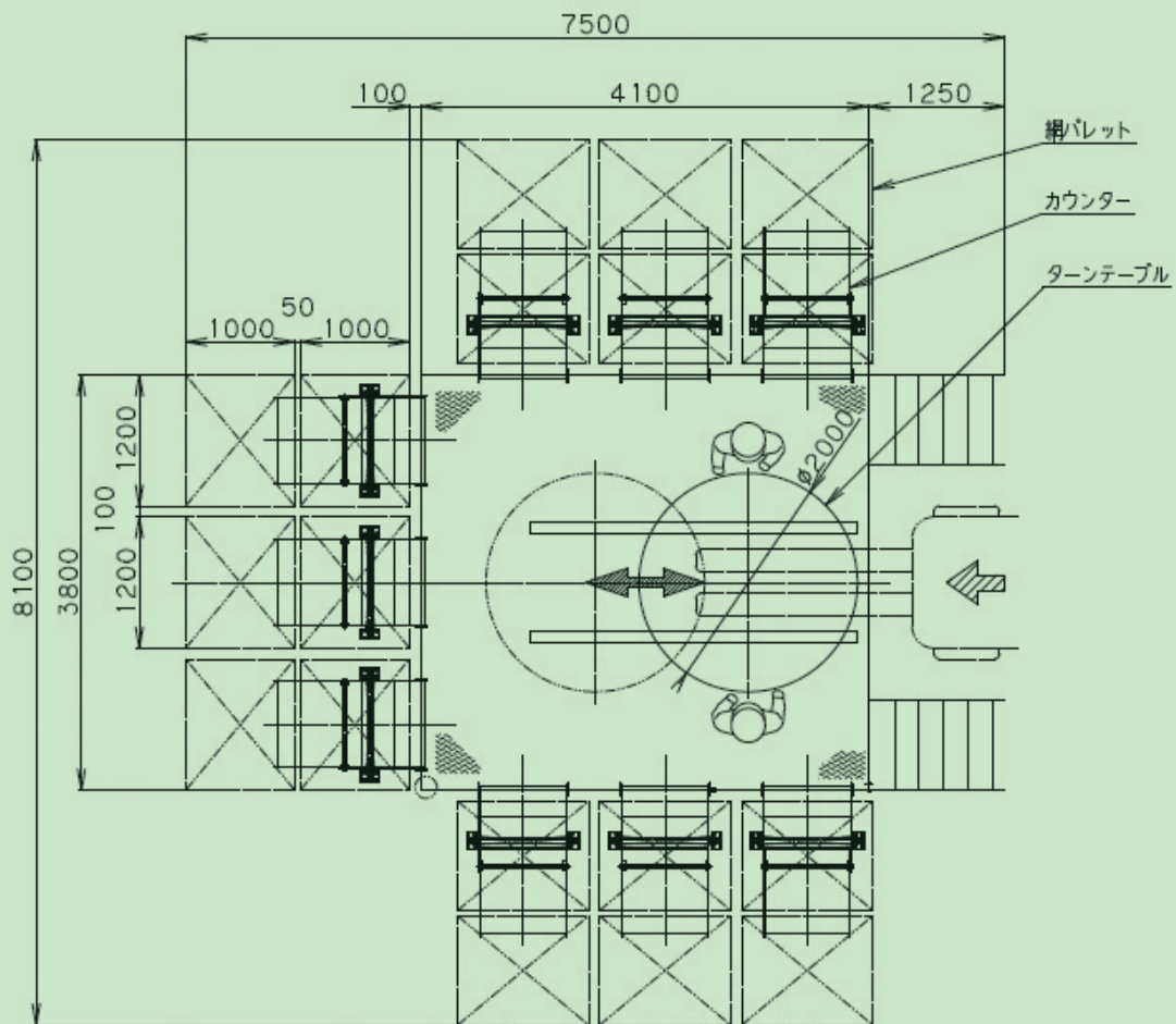
センターテーブル移動方式
