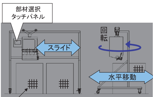
移動式カウンターイメージ(側面図)
