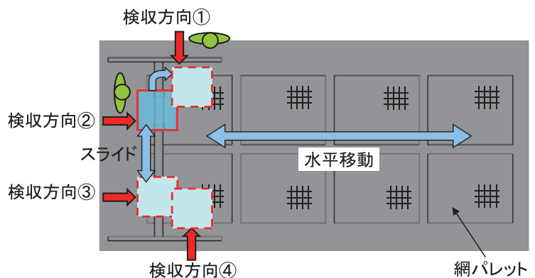
レイアウトイメージ(上面図)
